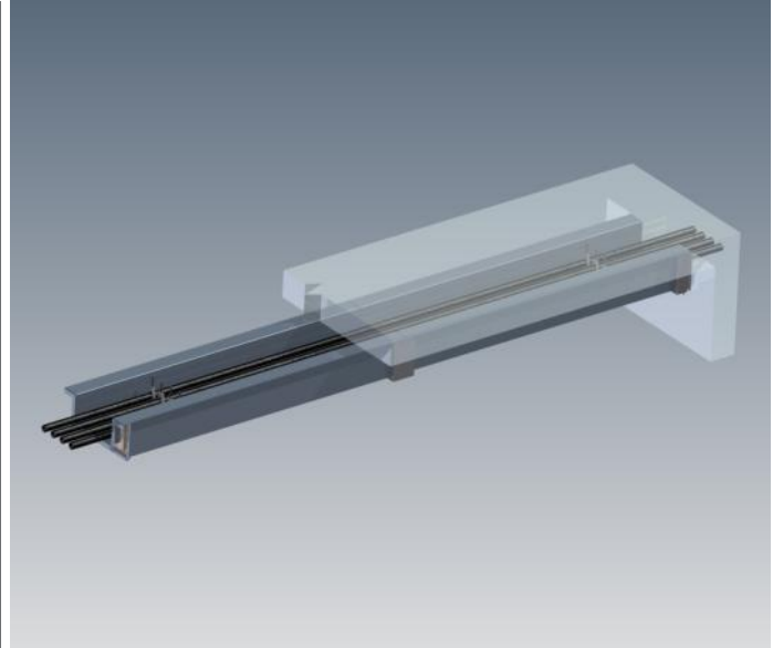
Rendu d'une enceinte pour tuyau à mazout.
