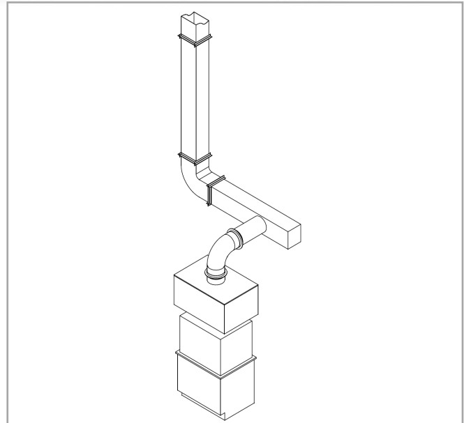
Imagen de un sistema de extracción para lavavajillas
